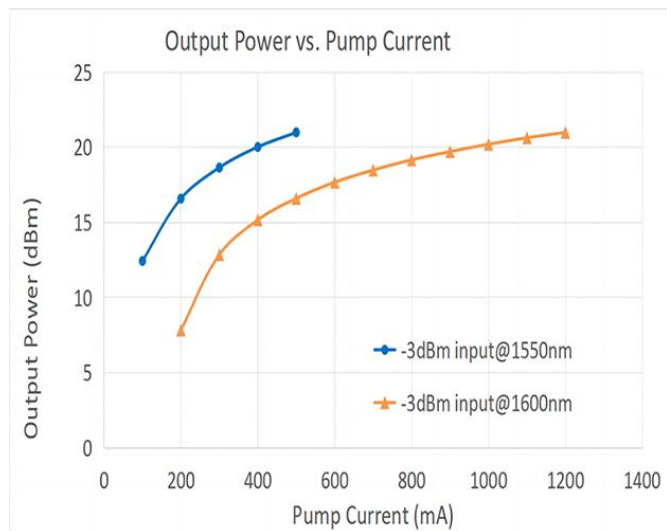
EDFA-CL-BA-20: 输出功率 vs 泵浦电流
