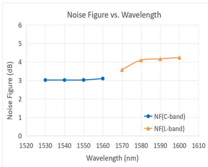
NF 噪声系数 EDFA-CL-BA-20: -3dBm 输入, 20dBm 输出
