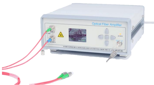
台式标准型模块尺寸: 260x280x120mm
