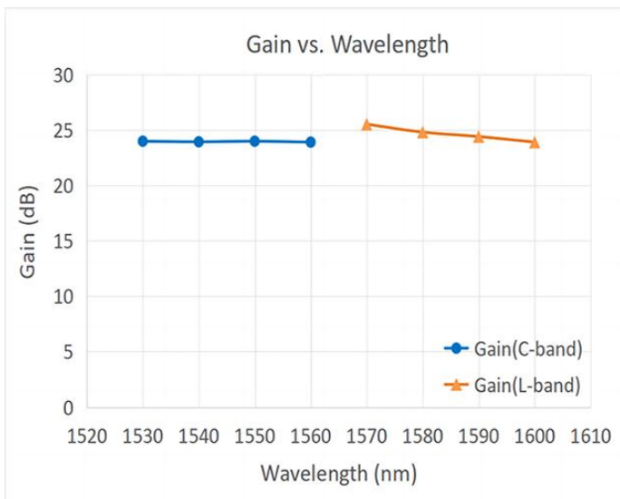
增益 EDFA-CL-BA-20: -3dBm 输入, 20dBm 输出
