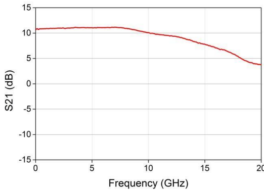
PD+频率响应曲线
