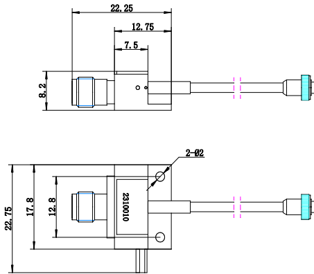
封装外形、尺寸及引脚定义 (单位: mm)
